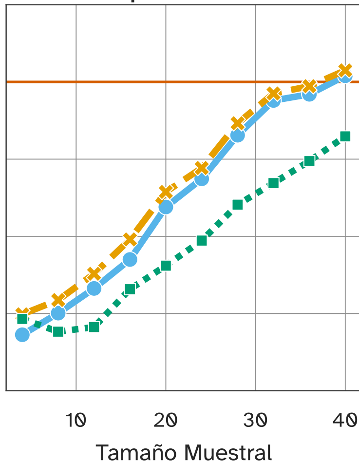
Exponencial
